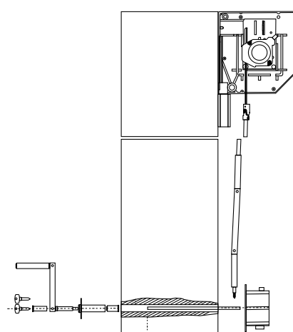
Manœuvre de secours extérieure-intérieure
