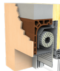
Pose en demi linteau maçonnerie
