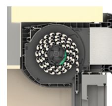
Pose en rénovation avec ITE*
