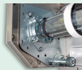
Joue acier sur silent-bloc Roulette souple anti-bruit
