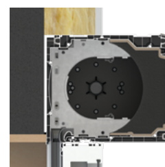
Pose en neuf
