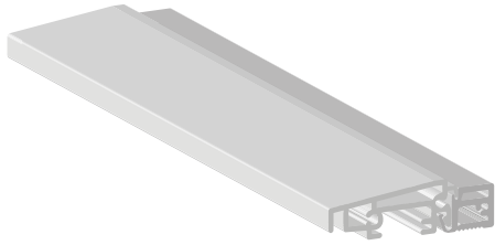
Aluminium anodisé argent Seuil plat 20 mm à rupture thermique Conforme PMR (Personnes à Mobilité Réduite)
