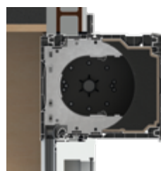
Pose en rénovation
