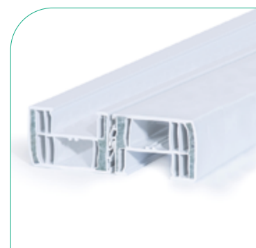
Renfort en fibres de verre
