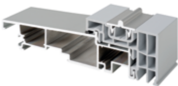
Seuil aluminium à rupture thermique
