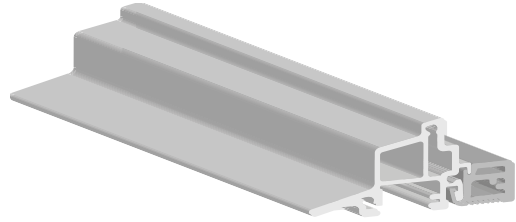
Aluminium anodisé argent Seuil 38 mm à rupture thermique
